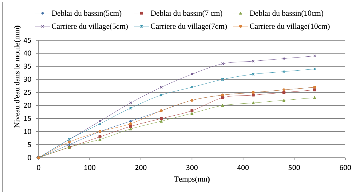
Figure 9 : Evolution de la vitesse d'infiltration des couches compactées
