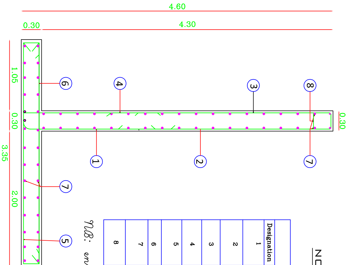
PLAN DE FERRAILLAGE
