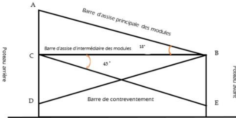
Figure 3 support métallique des modules.
