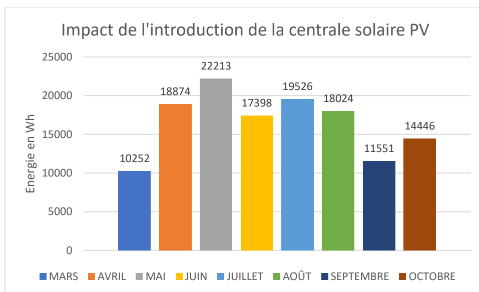
Figure 10 Différence de la consommation en énergie active après et avant l'implantation de la centrale
