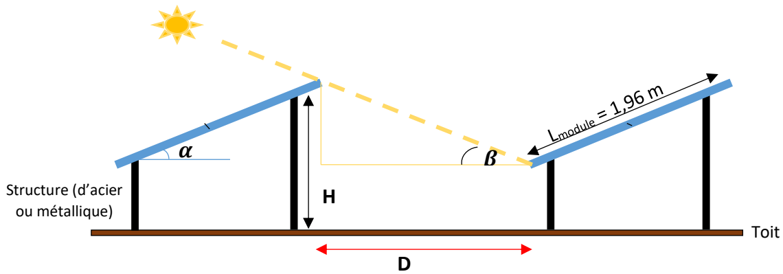
Figure 2 Illustration de l'ombrage dû aux modules.
