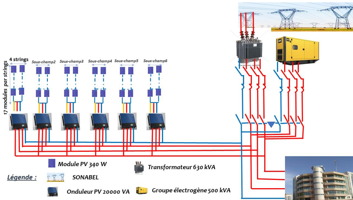
Figure 4 Schéma synoptique de la centrale
