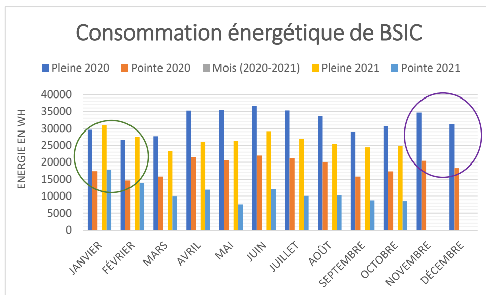
Figure 9 Consommation énergétique de BSIC 2020-2021
