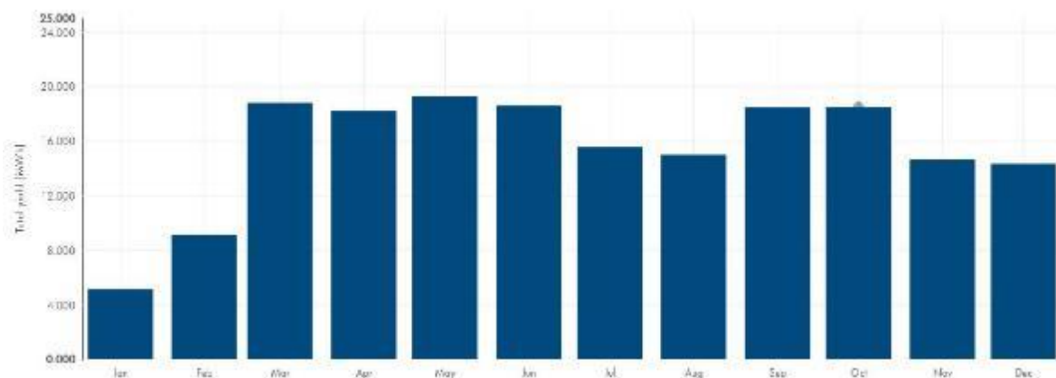
Figure 8 Production du champ solaire obtenu par data manager en MWh
