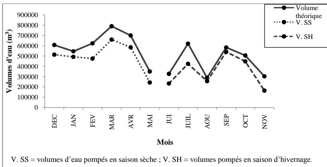
Figure 6 : Evolution des volumes d'eau calculés et ceux apportés aux parcelles
